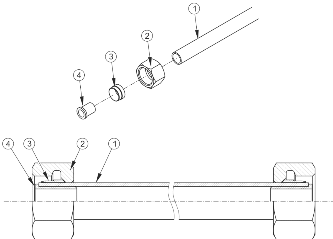
РИСУНОК 5.11 Монтаж пневмопровода
